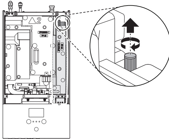
a Válvula tipo Schrader
